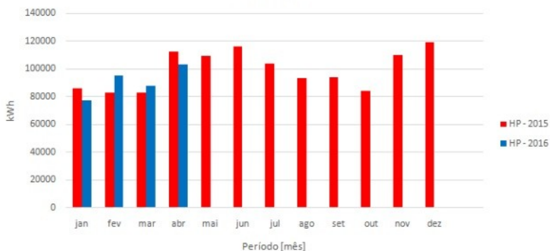
Comparação - Consumo 2015/2016 - Horário de Ponta 1215910-7
