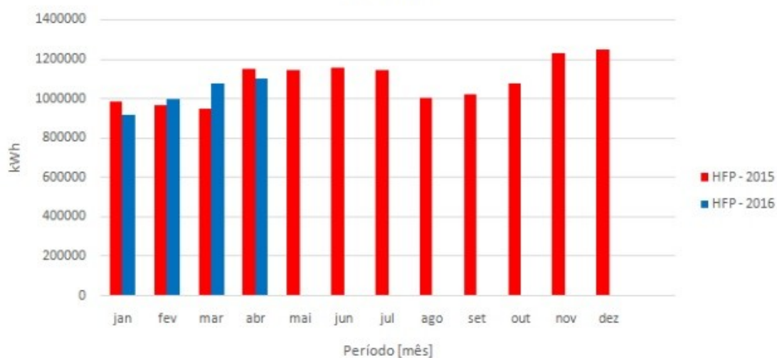
Comparação - Consumo 2015/2016 - Horário Fora de Ponta 1215910-7
